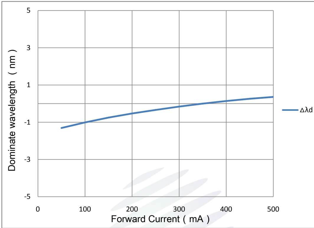
Fig. 1-12 Forward current vs. Dominant wavelength 主波长与正向电流特性曲线
