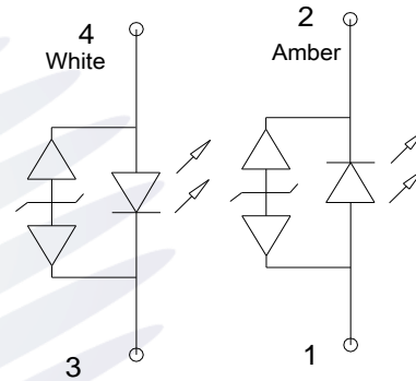
Fig.1-4 Polarity 极性
